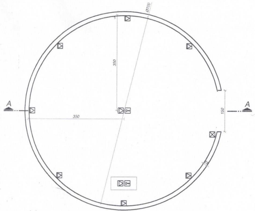
Planta Baixa Escala 1:50
